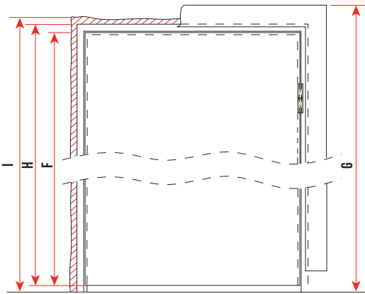
RESİM/PICTURE 2: KAPI YÜKSEKLİKLERİ/HEIGHT OF DOOR
